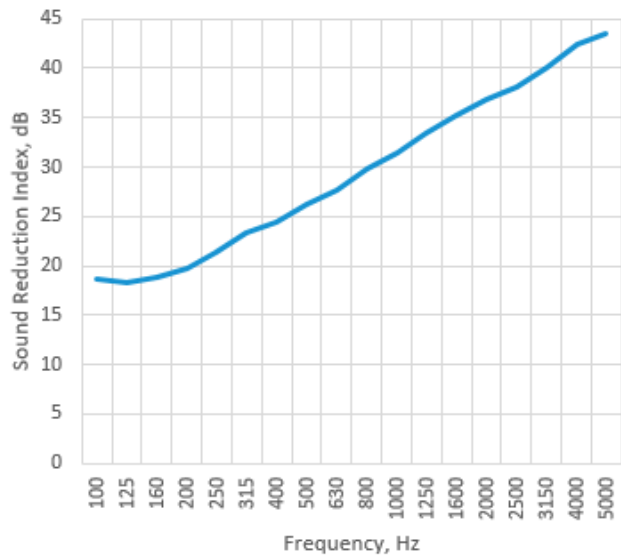
BS EN ISO 10140-2 Free Hanging Curtain
